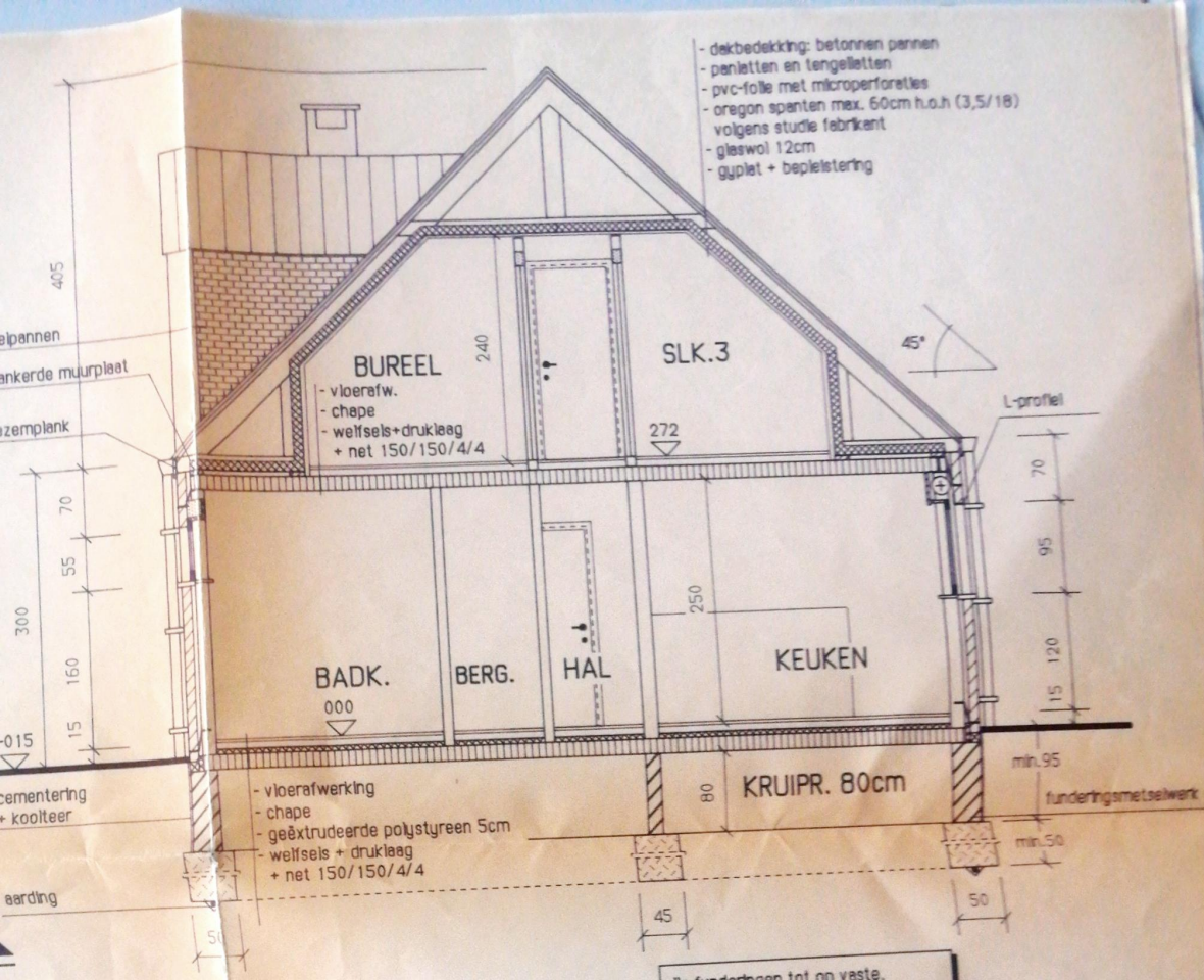
DOORSNEDE BB
