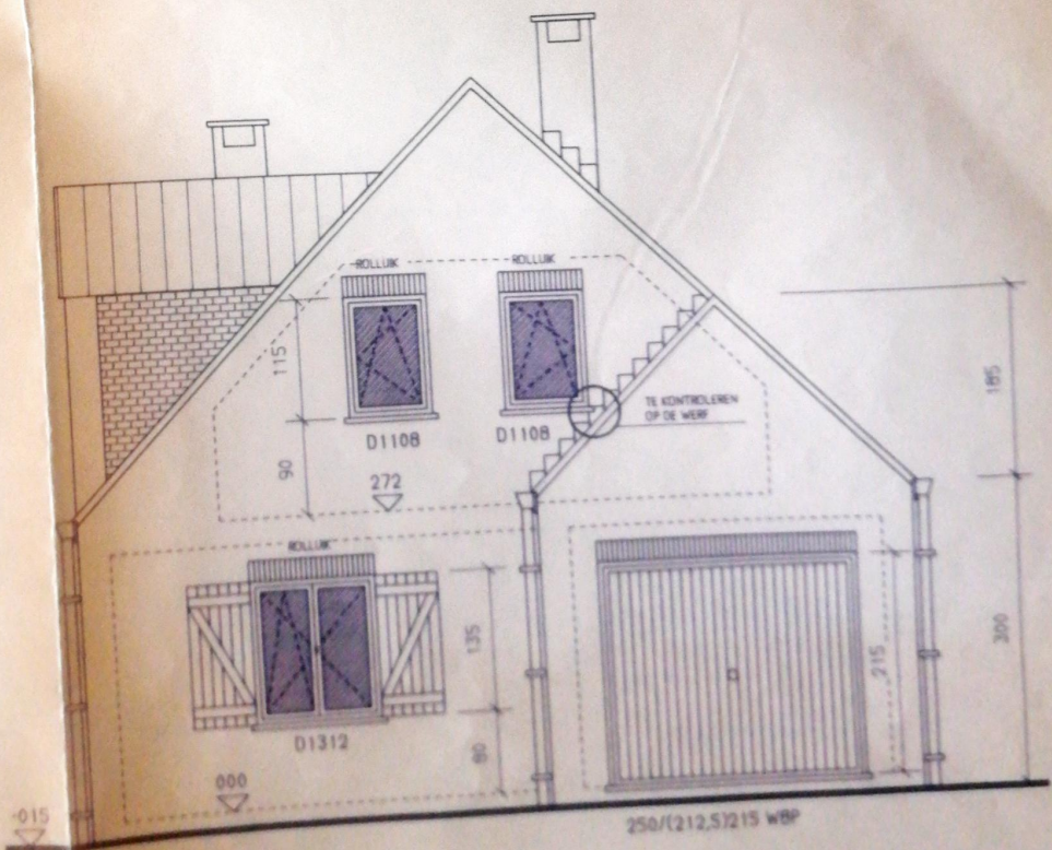
VOORGEVEL
